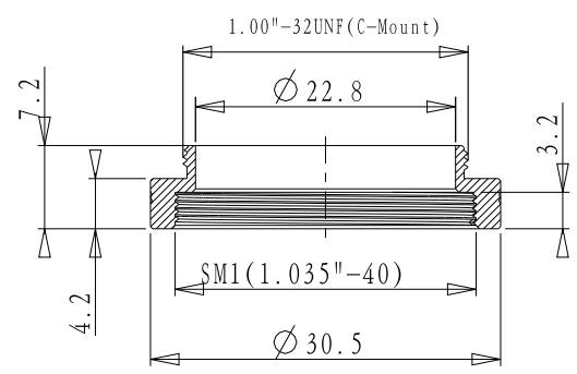
截面 A-A
