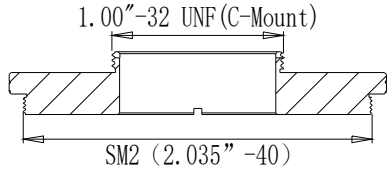
截面 A-A
