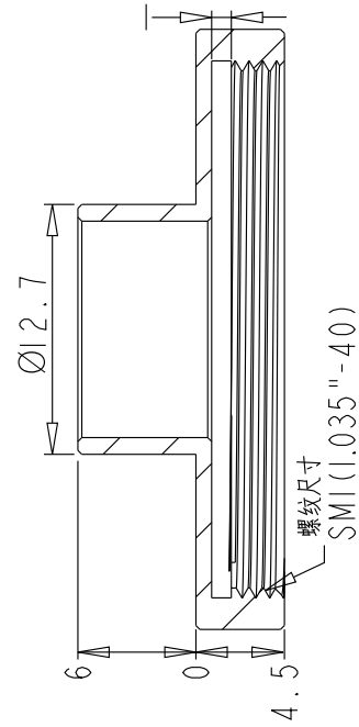
截面 A-A
