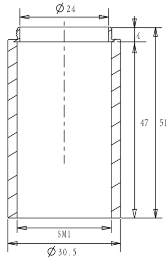
截面 A-A
