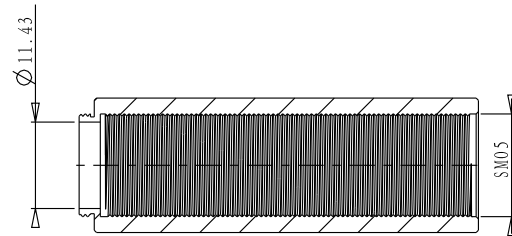
截面 A-A
