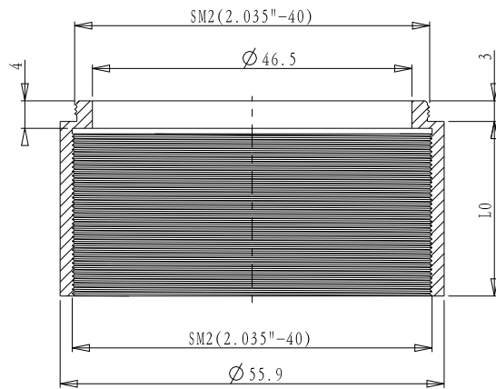
截面 A-A
