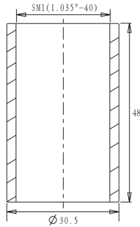
截面 A-A
