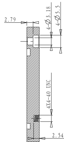
截面 B-B
