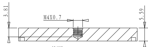
截面 A-A
