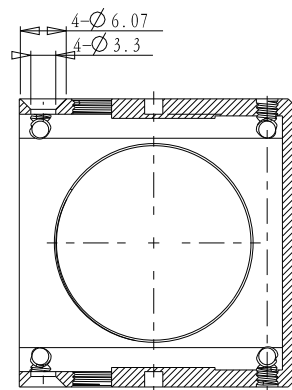
截面 A-A
