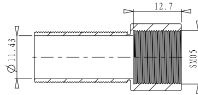
截面 A-A
