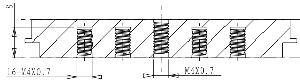
截面 A-A
