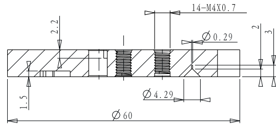
截面
