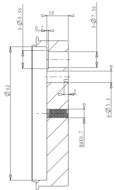
截面 A-A
