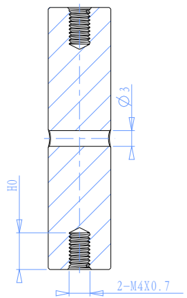
截面 A-A
