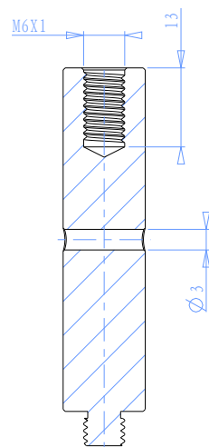
截面 A-A
