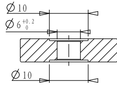
截面 A-A
