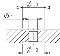
截面 A-A
