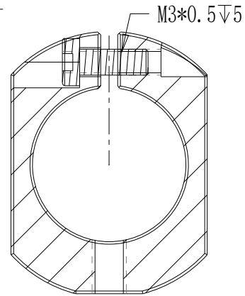
截面 A-A
