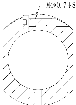
截面 A-A
