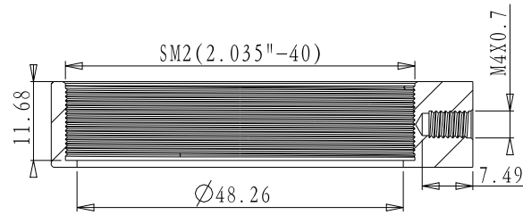
截面 A-A
