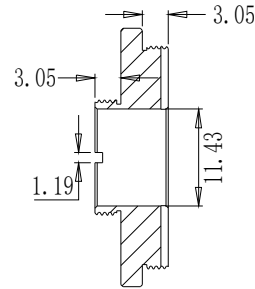
截面 A-A
