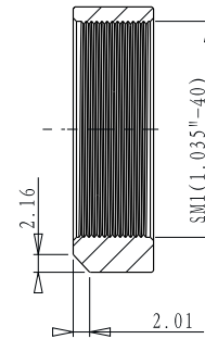
截面 A-A
